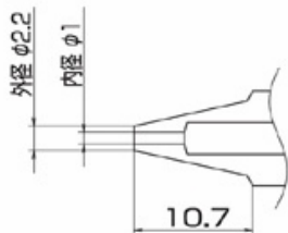
Düse N3 - 10 \phi 1,0mm
