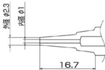
Düse N3 - L \phi 1,0mm lang
