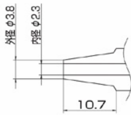
Düse N3Ø23 2,3mm
