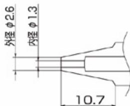
Düse N3 - 13 \phi 1,3mm
