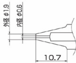
Düse N3 - 06 \phi 0,6mm
