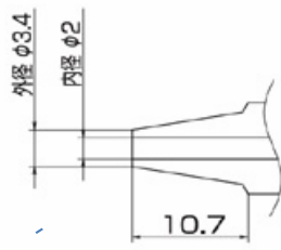
Düse N3 - 20 \phi 2,0mm
