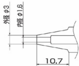
Düse NØ-16 1,6mm
