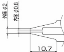
Düse N3 - 08 \phi 0,8mm
